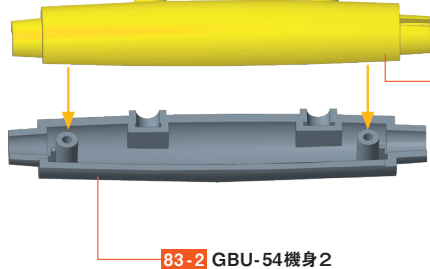
83-2 GBU-54機身2
